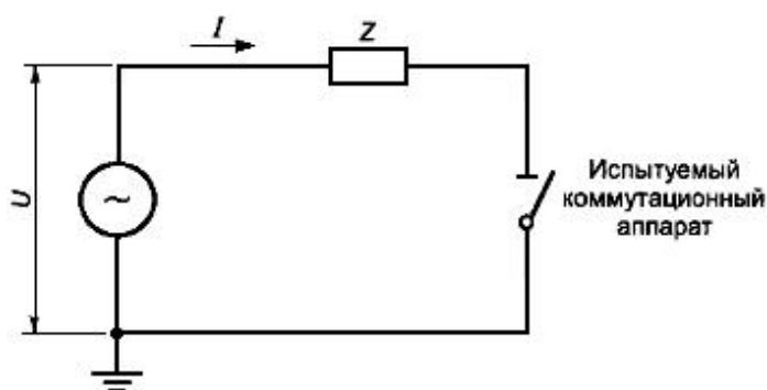
Схема А Испытуемый коммутационный аппарат
