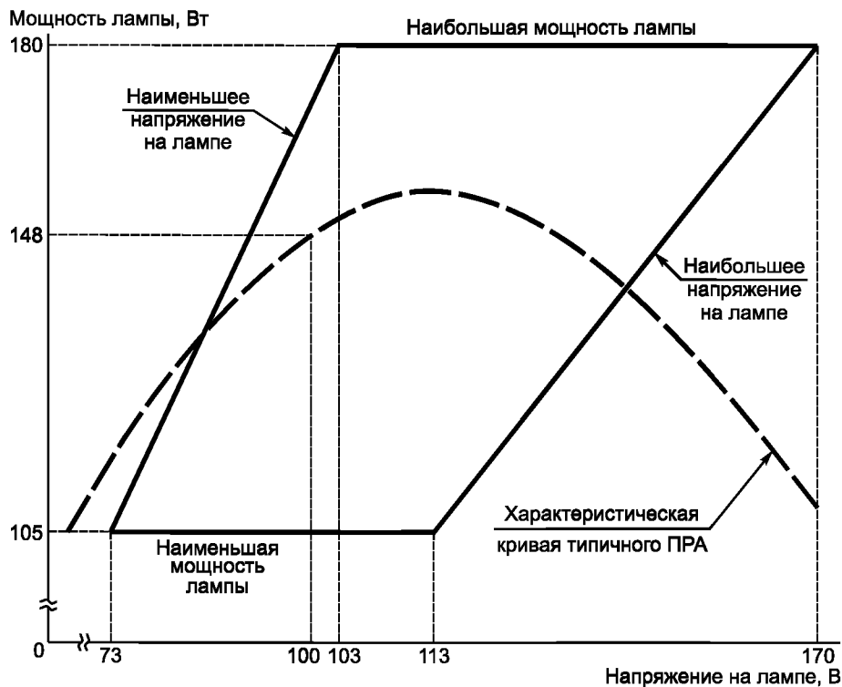
Рисунок Н.10 — Предельные рабочие характеристики ламп улучшенной цветности номинальной мощностью 150 Вт с прозрачной трубчатой или эллипсоидной с диффузным покрытием колбой
