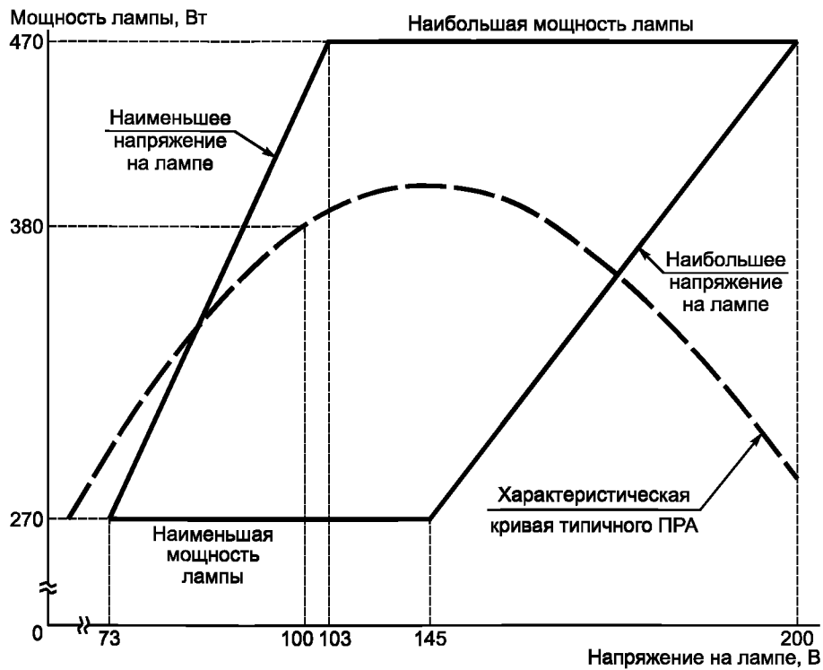
Рисунок Н.12 — Предельные рабочие характеристики ламп улучшенной цветности номинальной мощностью 400 Вт с прозрачной трубчатой колбой
