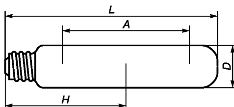
Рисунок В.1 — Лампа с трубчатой колбой
