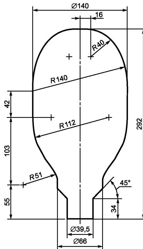
Рисунок G.4 — Эллипсоидная лампа мощностью 400 Вт
