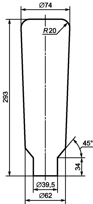
Рисунок G.3 — Трубчатая лампа мощностью 400 Вт
