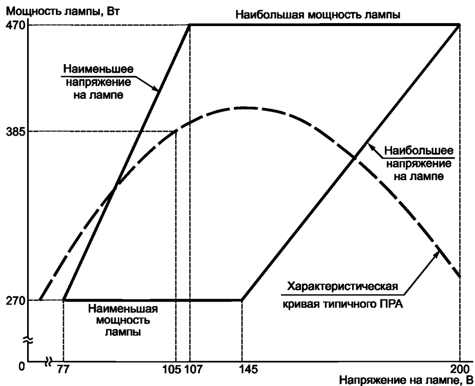
Рисунок Н.13 — Предельные рабочие характеристики ламп улучшенной цветности номинальной мощностью 400 Вт с эллипсоидной с диффузным покрытием колбой
