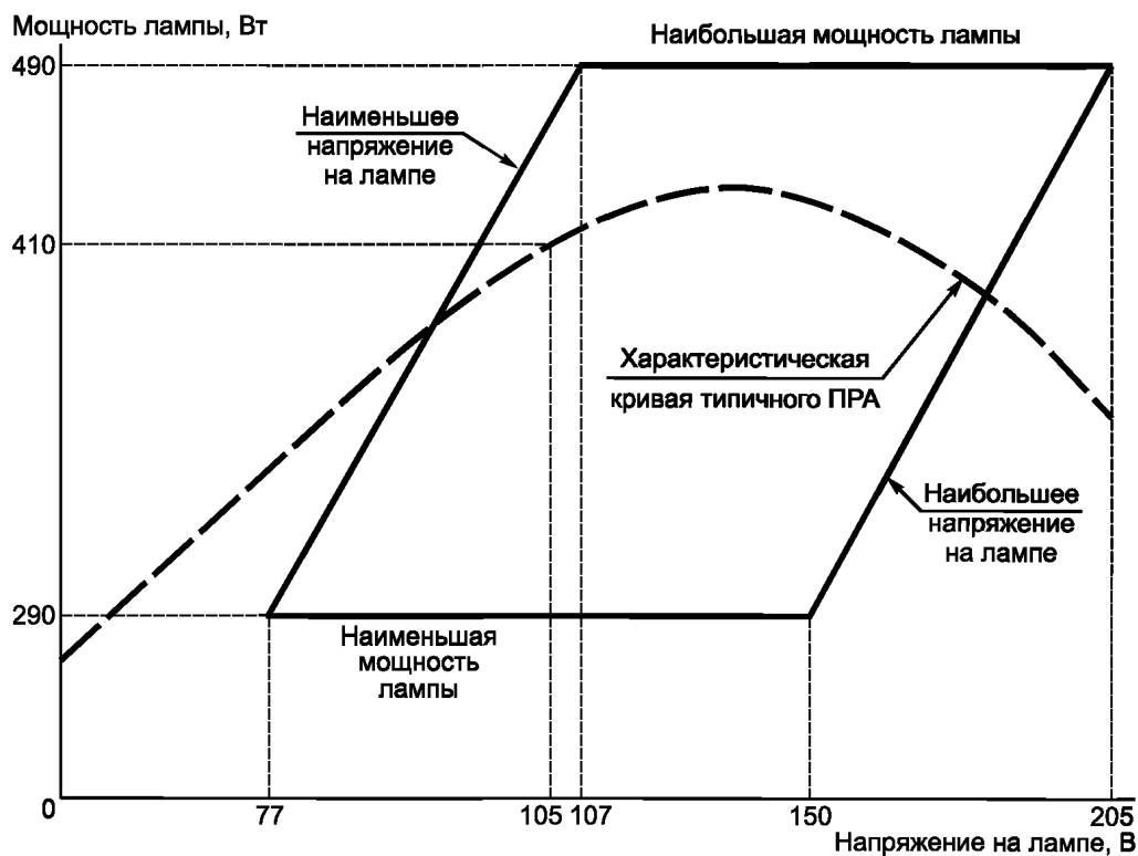
Рисунок Н.16 — Предельные рабочие характеристики ламп номинальной мощностью 400 Вт с повышенным напряжением зажигания, с эллипсоидной с диффузным покрытием колбой
