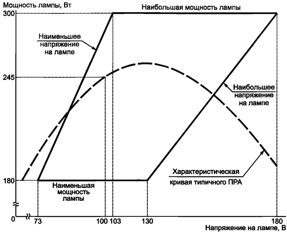
Рисунок Н.11 — Предельные рабочие характеристики ламп улучшенной цветности номинальной мощностью 250 Вт с прозрачной трубчатой или эллипсоидной с диффузным покрытием колбой
