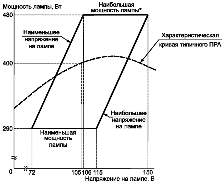
Рисунок Н.3 — Предельные рабочие характеристики ламп номинальной мощностью 400 Вт с эллипсоидной с диффузным покрытием колбой
