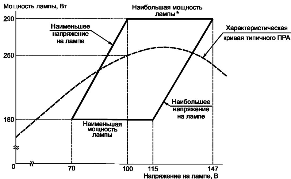
Рисунок Н.1 — Предельные рабочие характеристики ламп номинальной мощностью 250 Вт с прозрачной трубчатой или эллипсоидной с диффузным покрытием колбой
