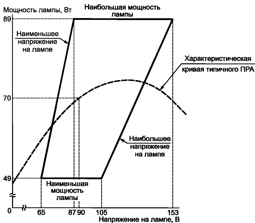
Рисунок Н.6 — Предельные рабочие характеристики ламп номинальной мощностью 70 Вт с прозрачной трубчатой, эллипсоидной прозрачной или с диффузным покрытием колбой
