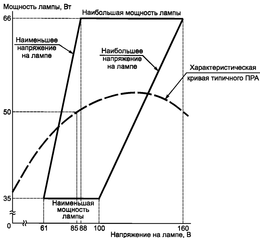
Рисунок Н.9 — Предельные рабочие характеристики ламп номинальной мощностью 50 Вт с трубчатой прозрачной, эллипсоидной прозрачной или с диффузным покрытием колбой
