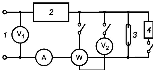
Рисунок Е.1 — Схема измерения параметров ламп
