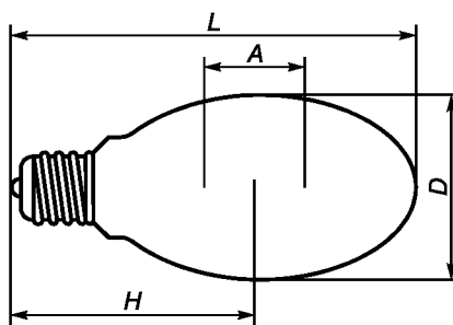
Рисунок В.2 — Лампа с эллипсоидной колбой
