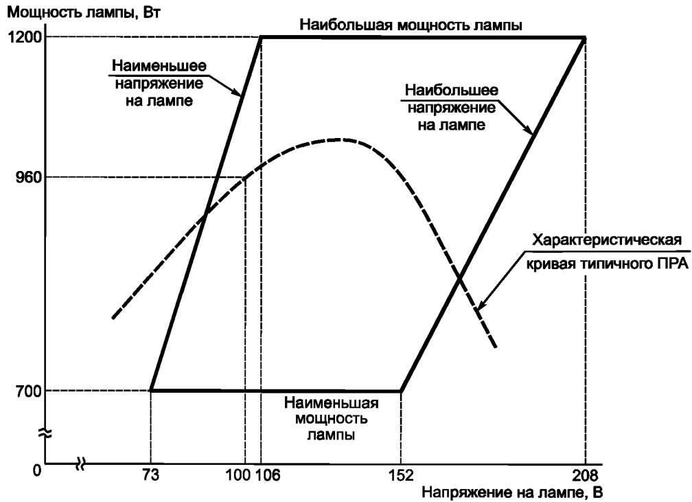
Рисунок Н.7 — Предельные рабочие характеристики ламп номинальной мощностью 1000 Вт с прозрачной трубчатой колбой
