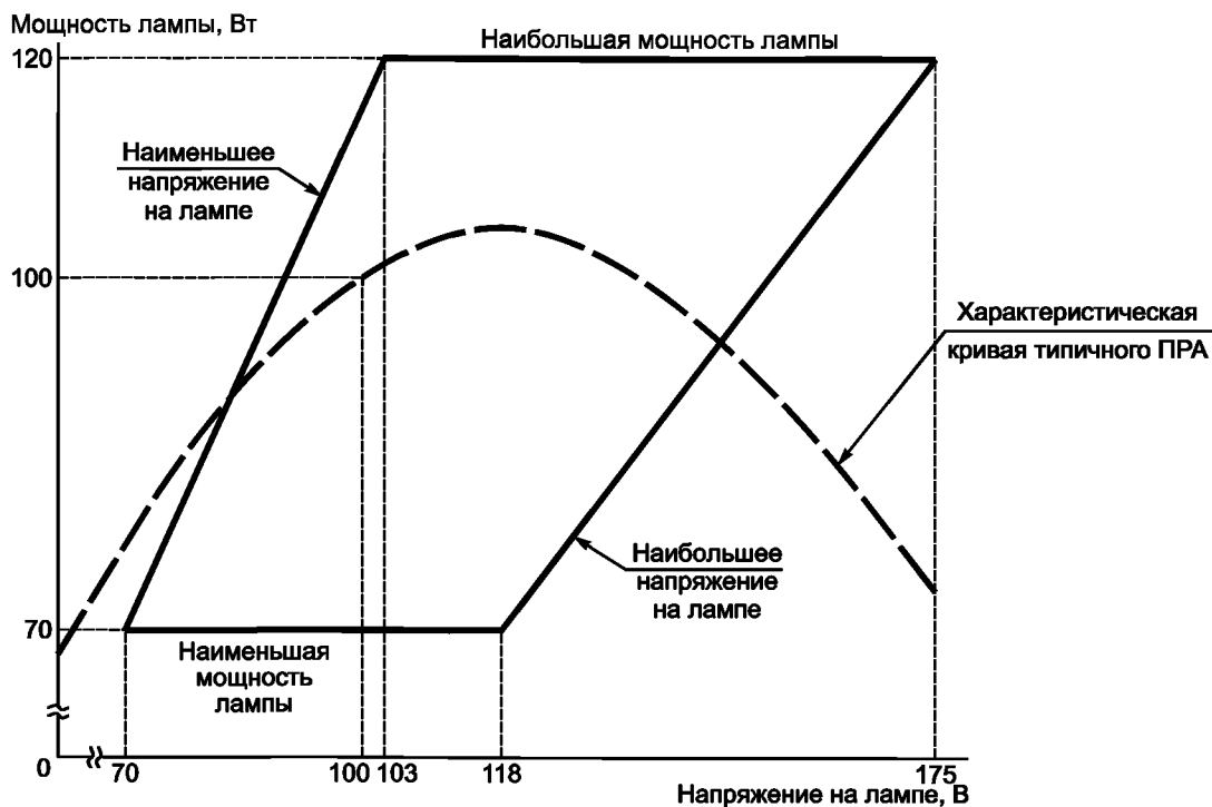
Рисунок Н.5 — Предельные рабочие характеристики ламп номинальной мощностью 100 Вт с трубчатой прозрачной или эллипсоидной с диффузным покрытием колбой
