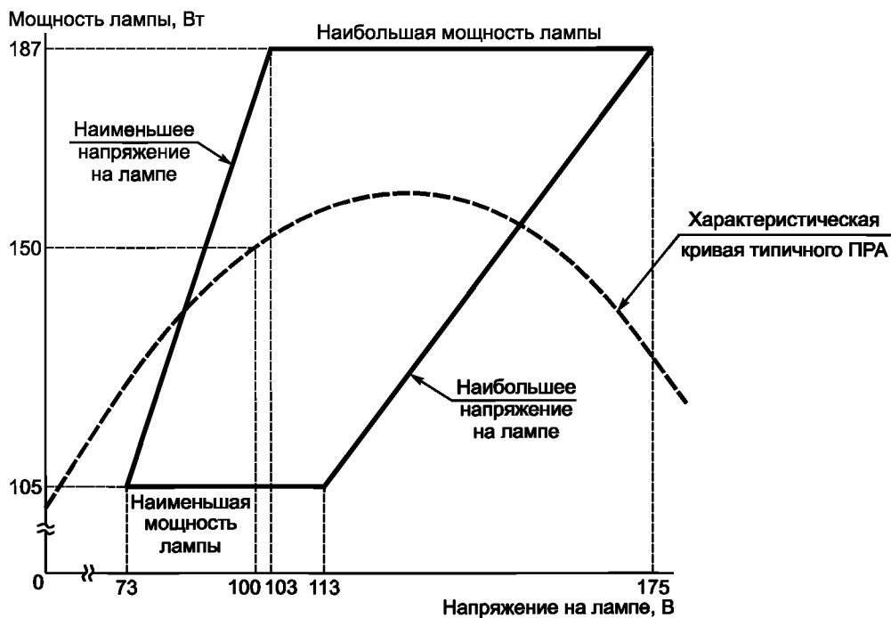
Рисунок Н.4 — Предельные рабочие характеристики ламп номинальной мощностью 150 Вт с прозрачной трубчатой или эллипсоидной с диффузным покрытием колбой
