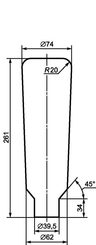
Рисунок G.1 — Трубчатая лампа мощностью 250 Вт
