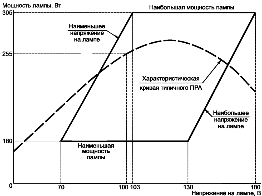
Рисунок Н.14 — Предельные рабочие характеристики ламп номинальной мощностью 250 Вт с повышенным напряжением зажигания, с прозрачной трубчатой или эллипсоидной с диффузным покрытием колбой
