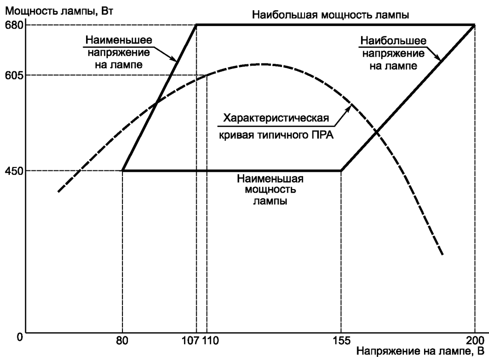
Рисунок Н.17 — Предельные рабочие характеристики ламп номинальной мощностью 600 Вт с трубчатой прозрачной колбой
