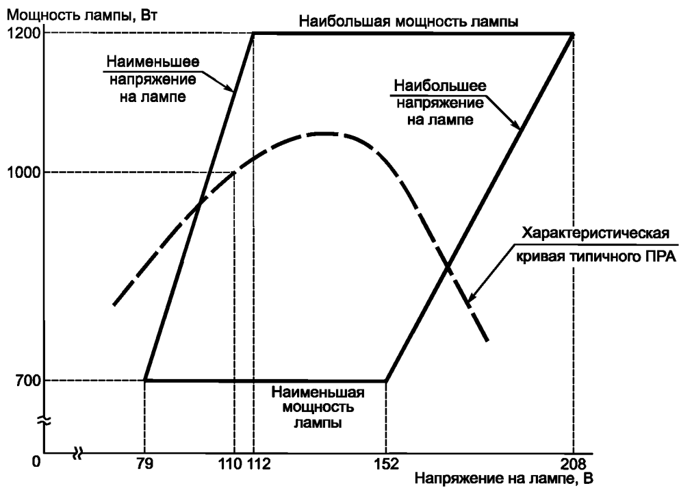
Рисунок Н.8 — Предельные рабочие характеристики ламп номинальной мощностью 1000 Вт с эллипсоидной с диффузным покрытием колбой
