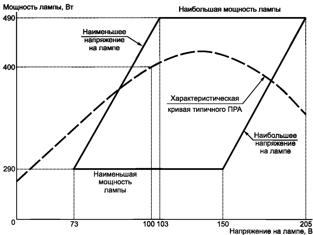
Рисунок Н.15 — Предельные рабочие характеристики ламп номинальной мощностью 400 Вт с повышенным напряжением зажигания, с прозрачной трубчатой колбой
