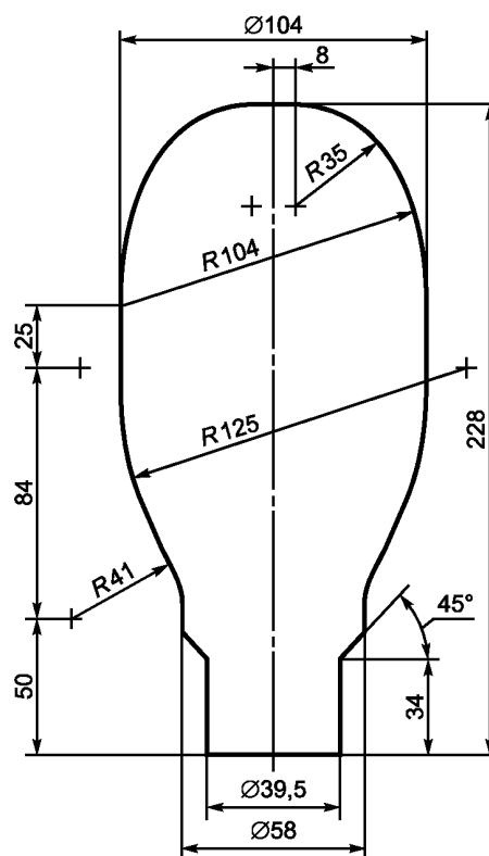
Рисунок G.2 — Эллипсоидная лампа мощностью 250 Вт
