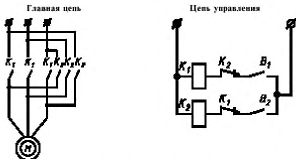
K_1 и K_2 — испытуемые пускатели, M — заторможенный двигатель
