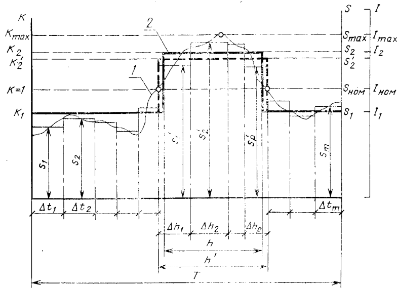
1—исходный график нагрузки; 2—двухступенчатый прямоугольный график нагрузки
